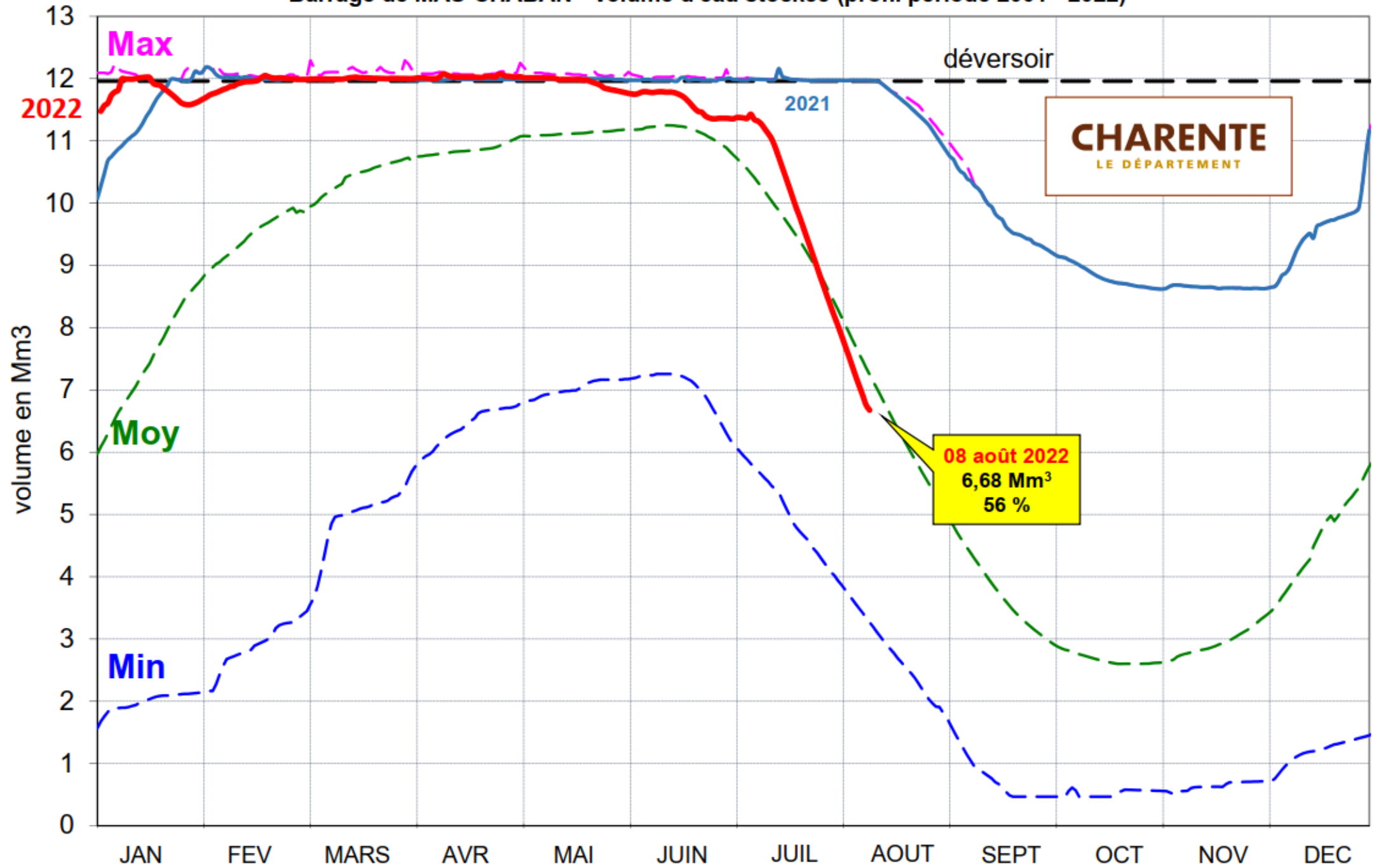
Barrage de MAS-CHABAN - Volume d'eau stockée (profil période 2001 - 2022)
